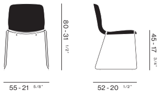
ALFA 4 pieds ALFA 4 patas
