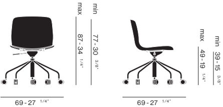
ALFA 5 branches en aluminium “Office” ALFA 5 radios de acero “Office”
