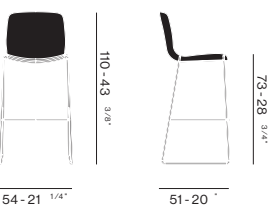
ALFA tabouret piètement traineau ALFA taburete patin
