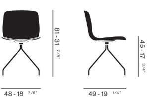
ALFA piètement tréteau fixe “Classic” ALFA estructura fija “Classic”
