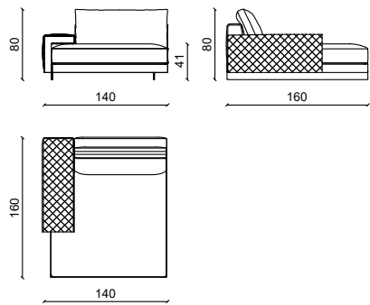
ELEMENTO / ELEMENT 260
