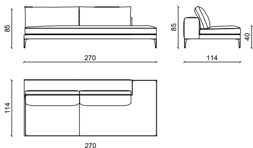
ELEMENTO / ELEMENT 270
