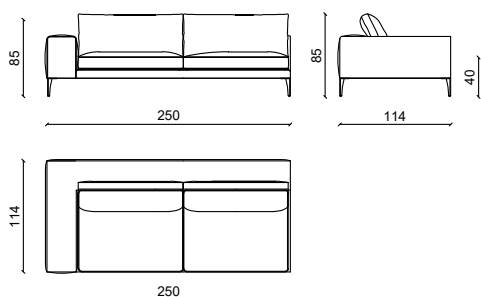
ELEMENTO / ELEMEN 250
