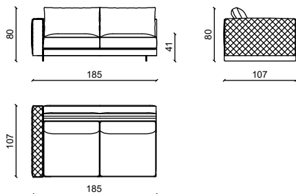
ELEMENTO / ELEMENT 185
