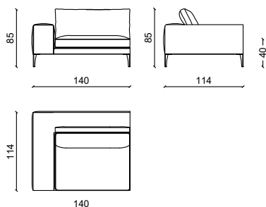
ELEMENTO / ELEMENT 140
