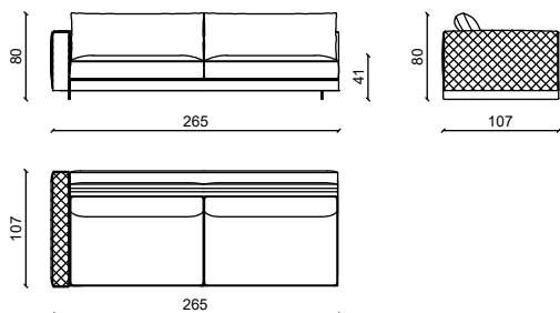
ELEMENTO / ELEMENT 265
