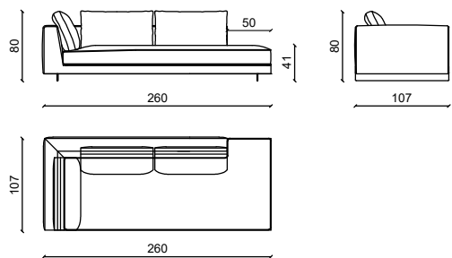
ELEMENTO / ELEMENT 260
